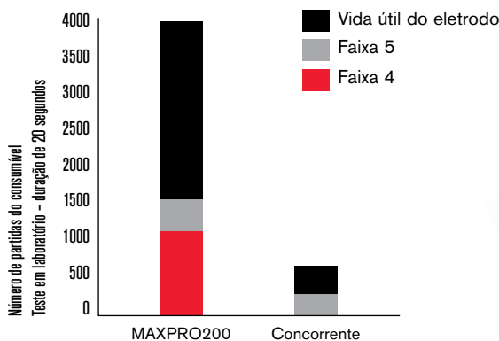
MAXPRO200 Tocha manual de 65°
